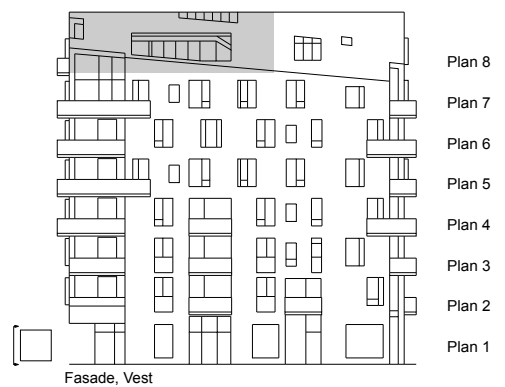
Fasade, Vest
